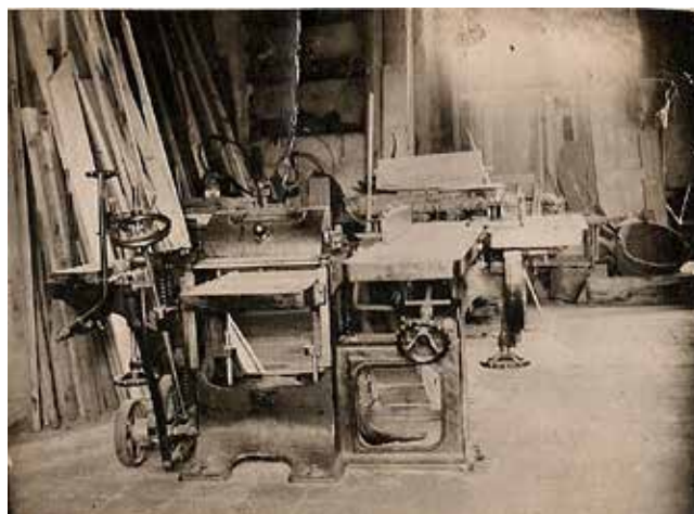
Interior de la fusteria. La màquina combinada per planejar, regruixar, serrar i motllurar i fer forats. Va ser utilitzada fins els anys 70.
